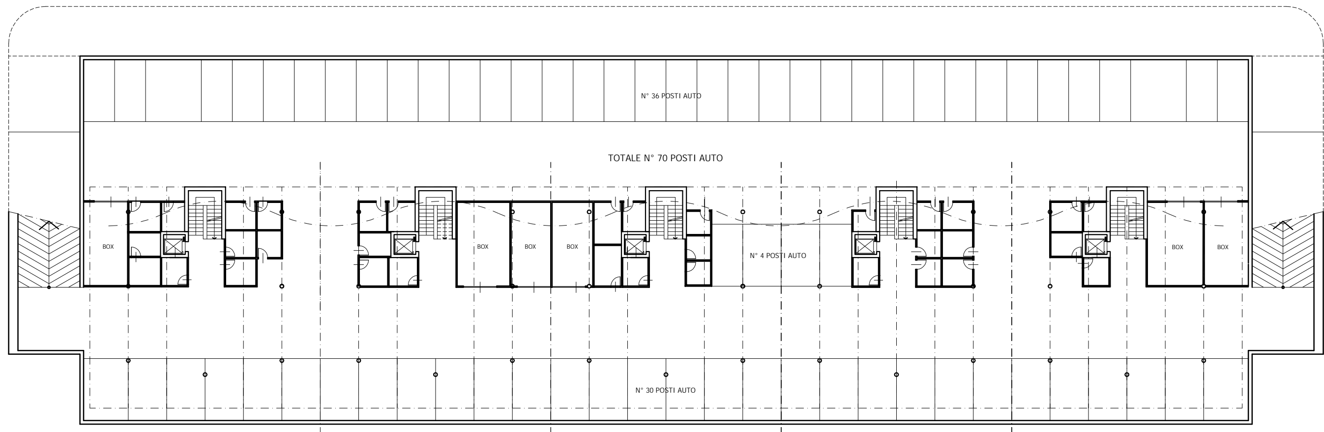
PIANTA PIANO INTERRATO sc. 1:300
