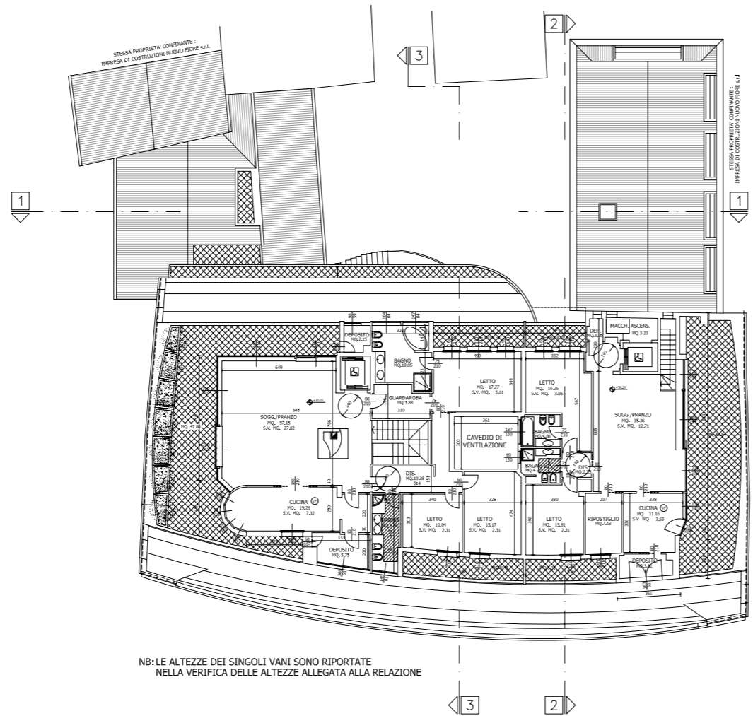
PIANTA LIVELLO 7 (Q.+30.55)
