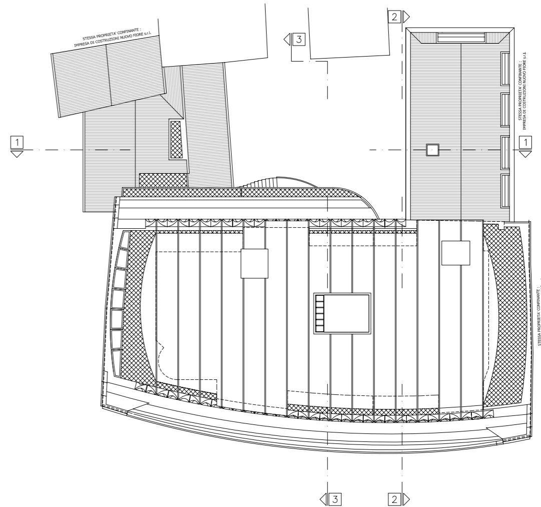
PIANTA LIVELLO 8 COPERTURA
