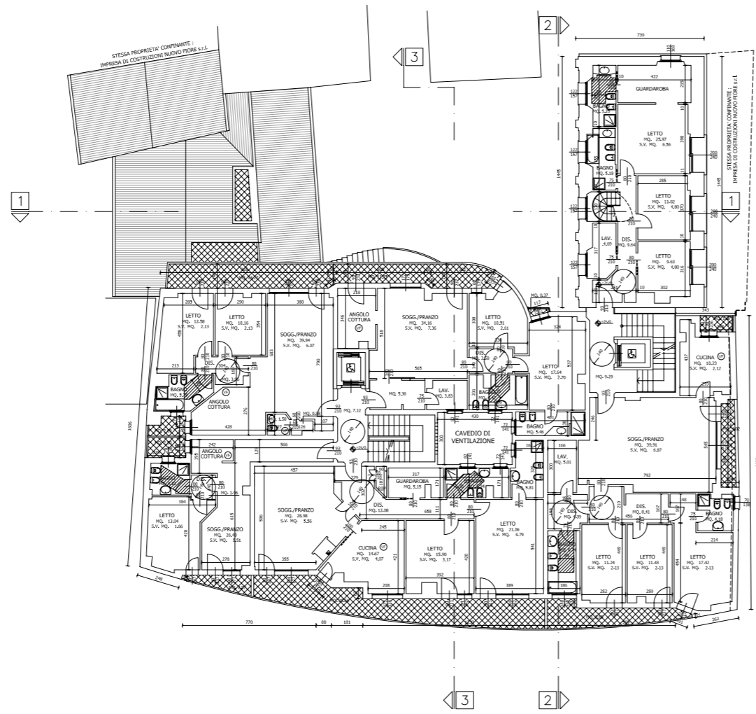
PIANTA LIVELLO 5 (Q.+24.45)
