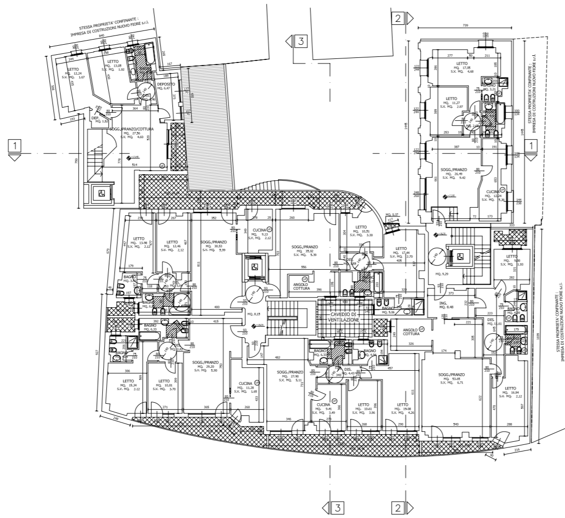
PIANTA LIVELLO 3 (Q.+18.35)
