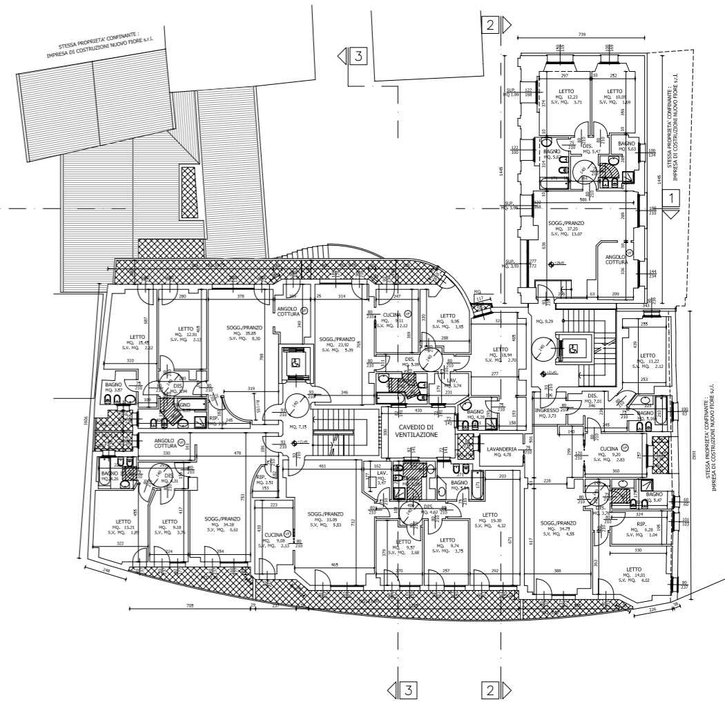
PIANTA LIVELLO 4 (Q.+21.40)
