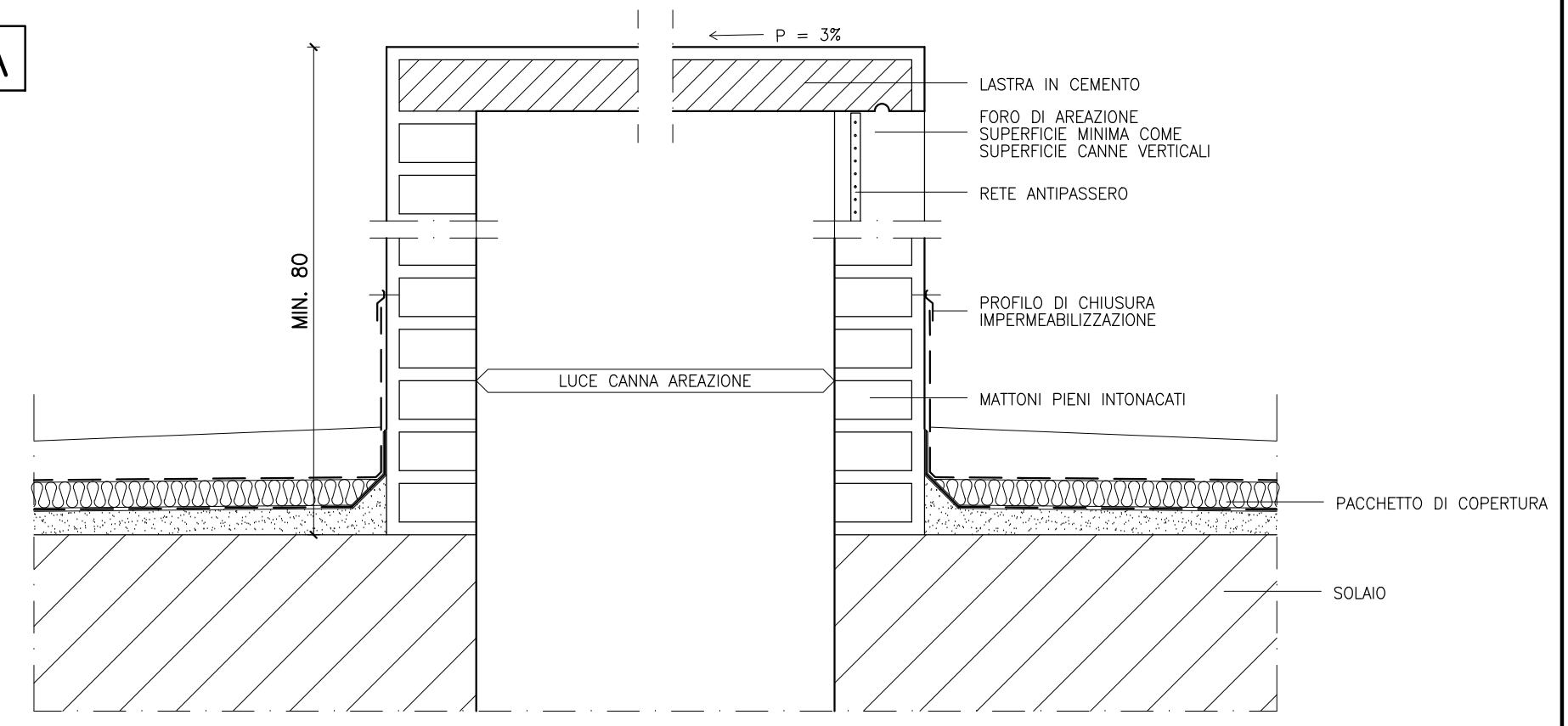
PARTICOLARE COMIGNOLO CANNE VENTILAZIONE SC.1:10
