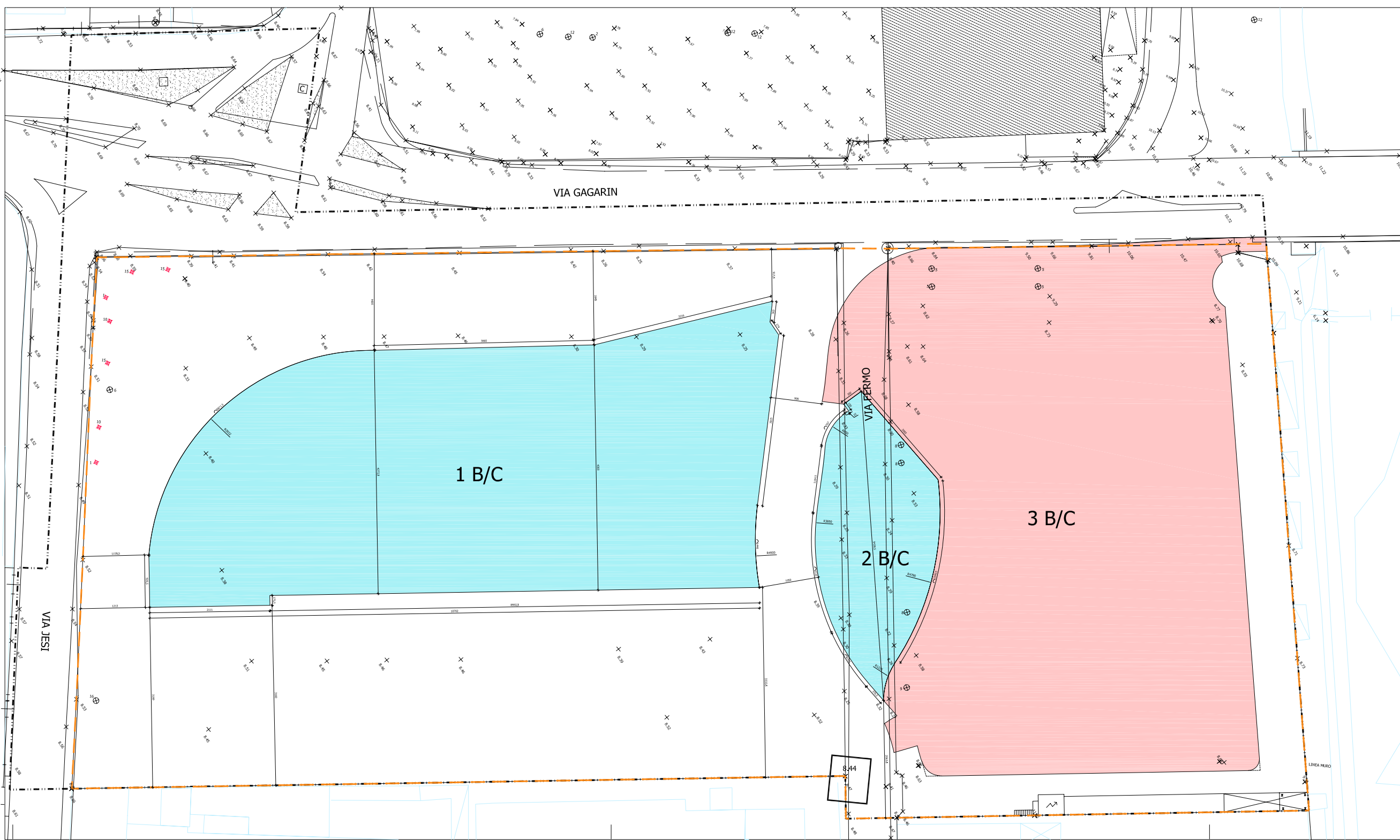
RILIEVO PLANOALTIMETRICO DELLO STATO DI FATTO Scala 1:200
